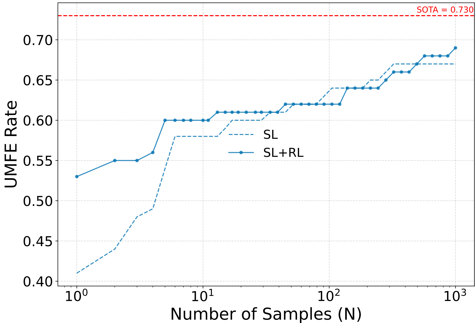
Best-of-N UMFE Rate
