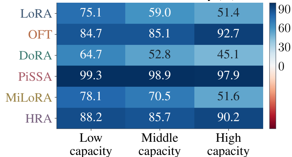
Llama-8B: NLL recovery (%)
