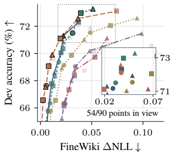
(b) Llama-3.1-8B
