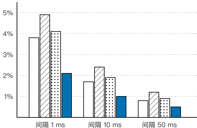
E1000e: netperf TCP_RR 吞吐降低
