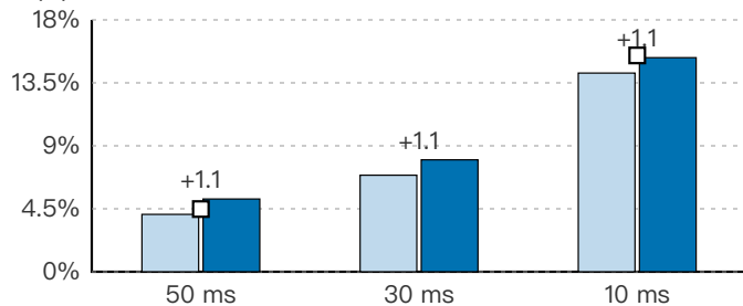
(b) virtio-net UDP
