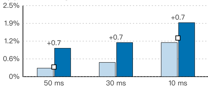
(d) virtio-scsi 写
