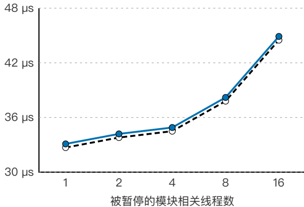
(b) 单次随机化的迁移时间随被暂停线程数
