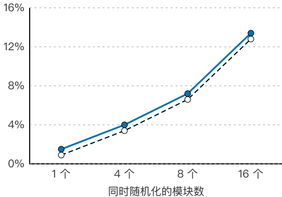
(a) CPU 开销随同时随机化的模块数 (50 ms 间隔)
