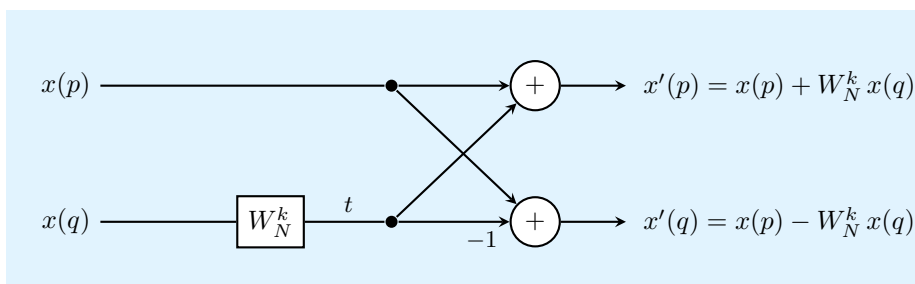
Rysunek 3.1: Operacja motylkowa (ang. butterfly ) algorytmu FFT o podstawie 2, opracowanie własne na podstawie [?]
