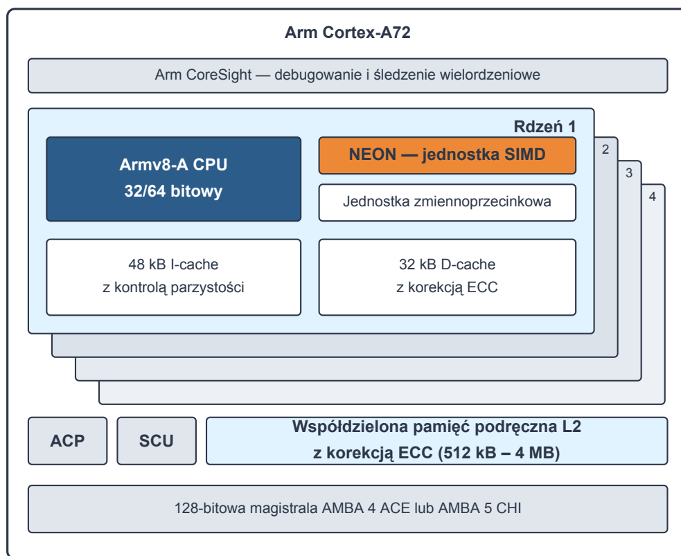
Rysunek 4.1: Uproszczony schemat rdzenia Cortex-A72 z zaznaczoną jednostką NEON. Opracowanie własne na podstawie [? ].
