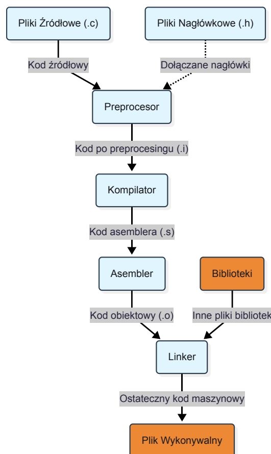
Rysunek 3.4: Klasyczny przebieg systemu przetwarzania języka programowania [? ]
