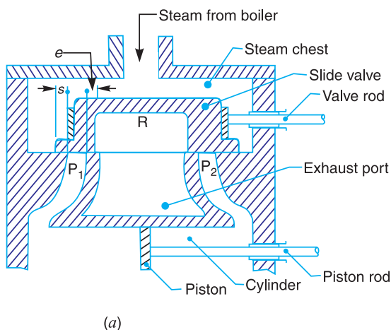
Fig. 17.2. D -slide valve.
