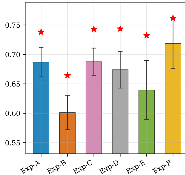
F1
