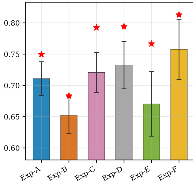
Precision
