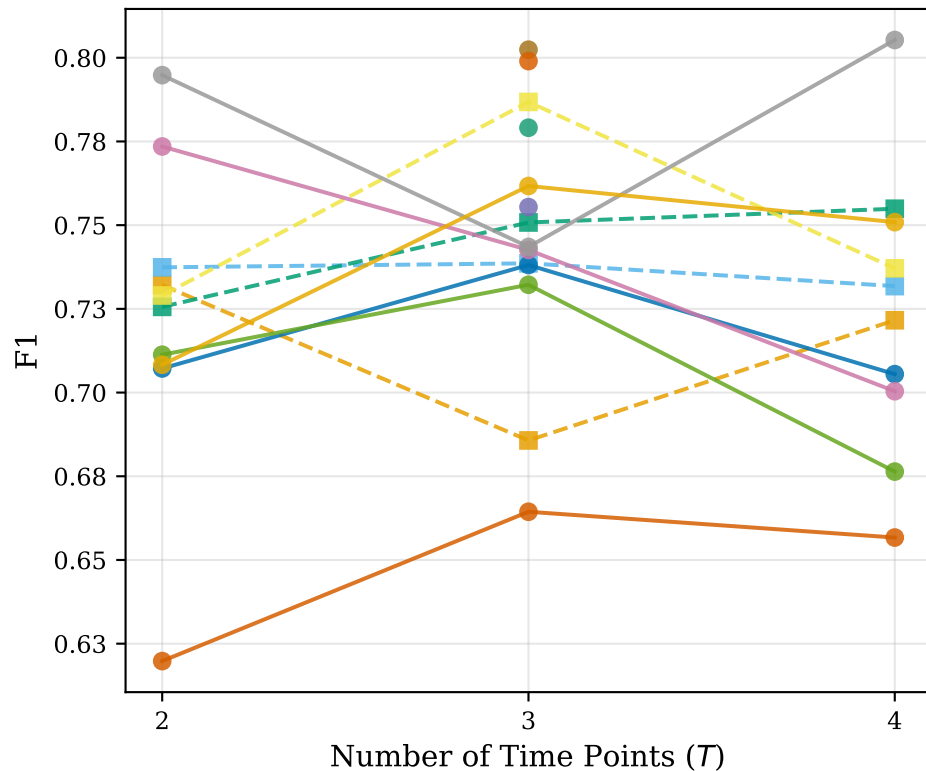
Best F1 vs. Temporal Resolution
