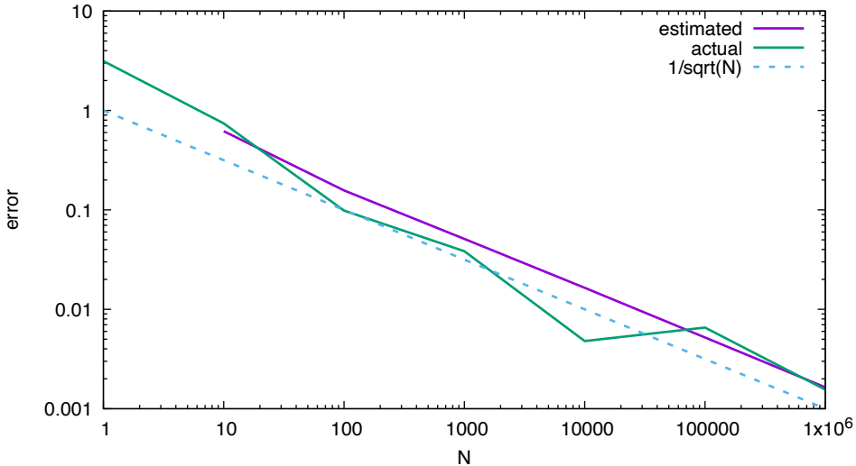
Monte Carlo error scaling
