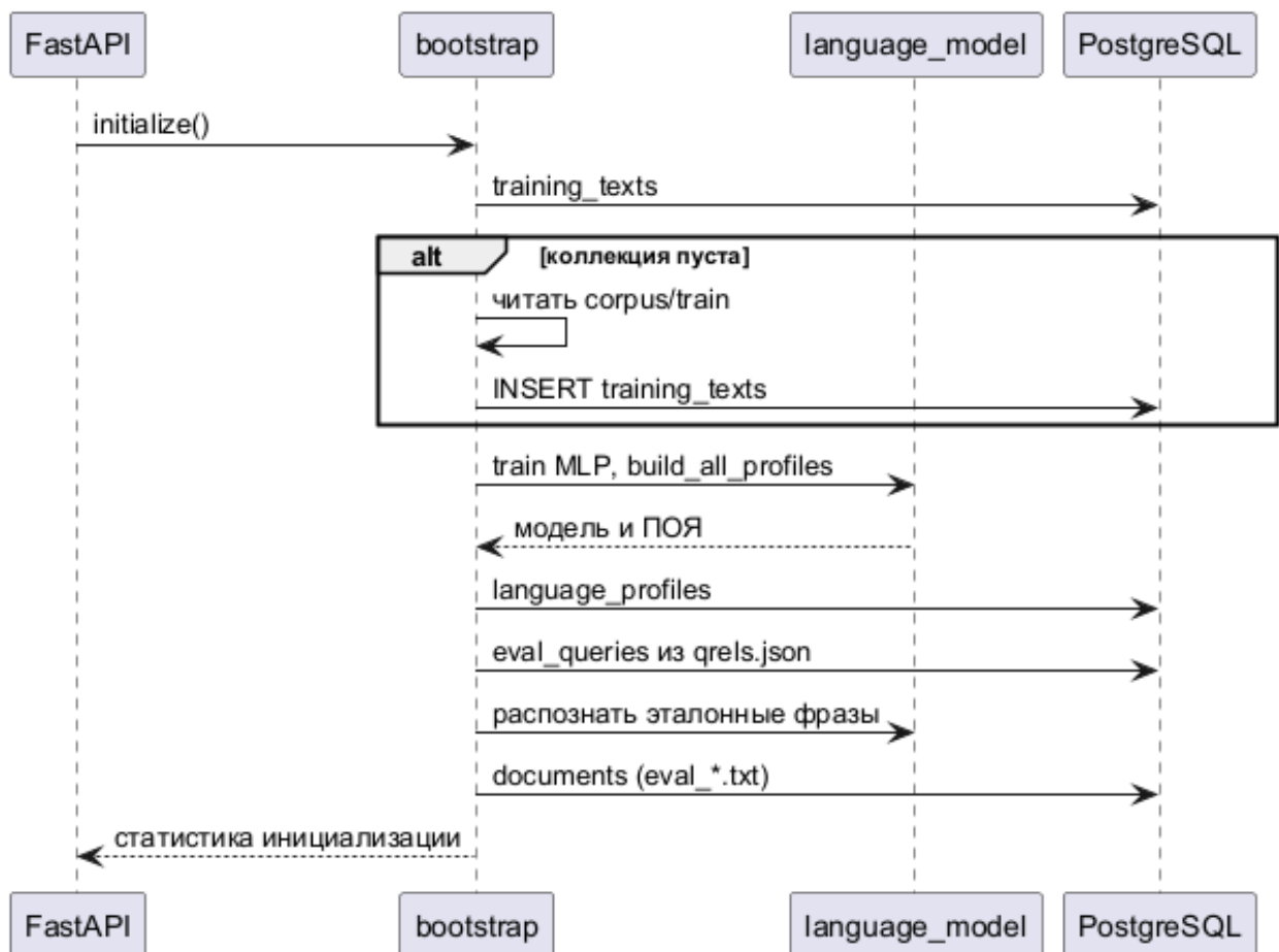
Рисунок 2.2 – Обучение моделей при запуске сервера.
