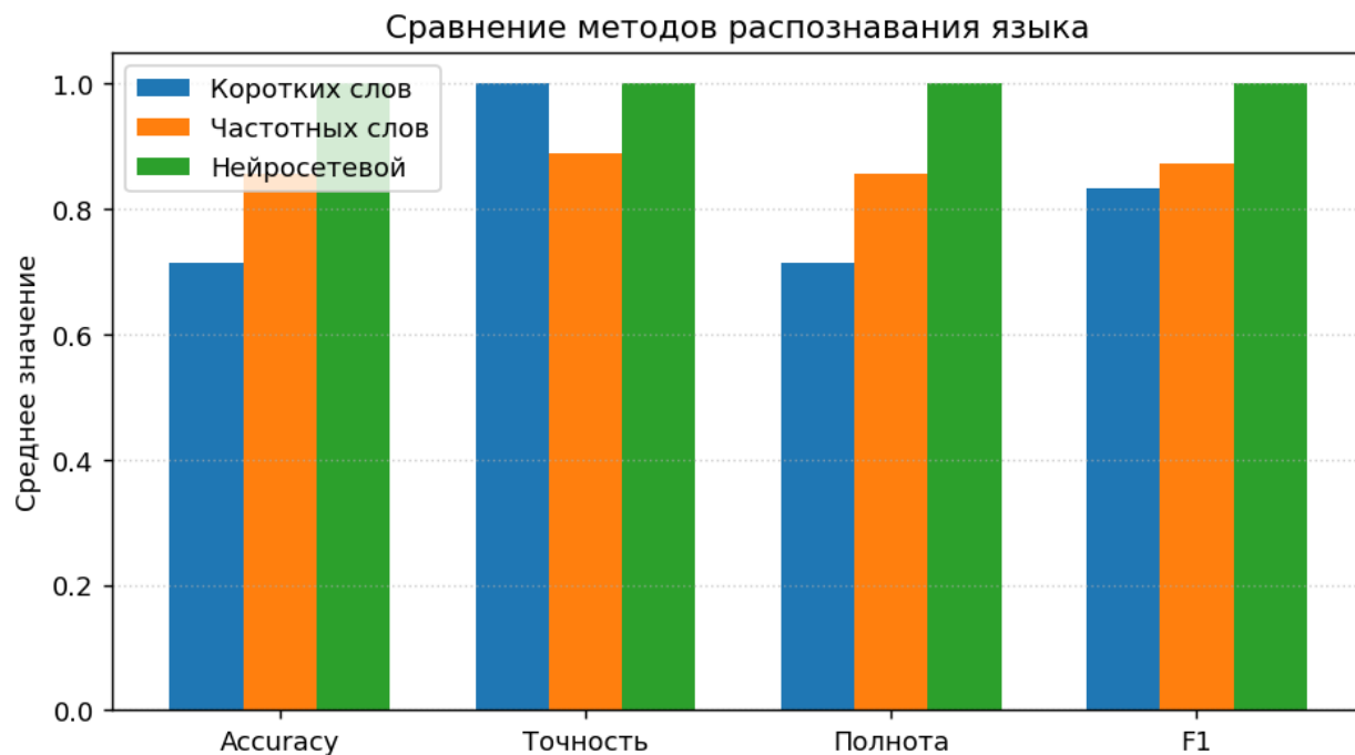
Рисунок 2.5 – Сравнение методов по качеству.
