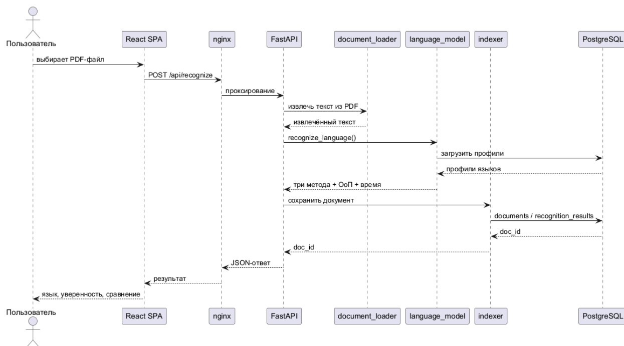
Рисунок 2.3 – Распознавание загруженного PDF.
