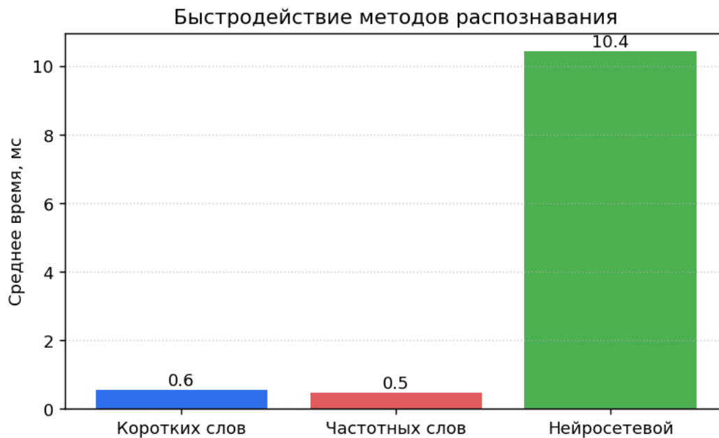
Рисунок 2.6 – Среднее время на проверочных фразах.
