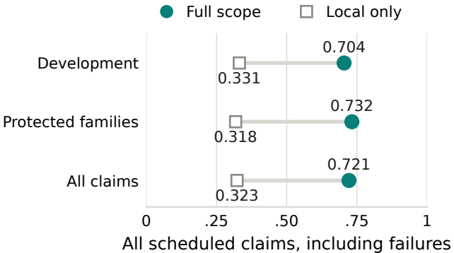
Reference-chain precision
