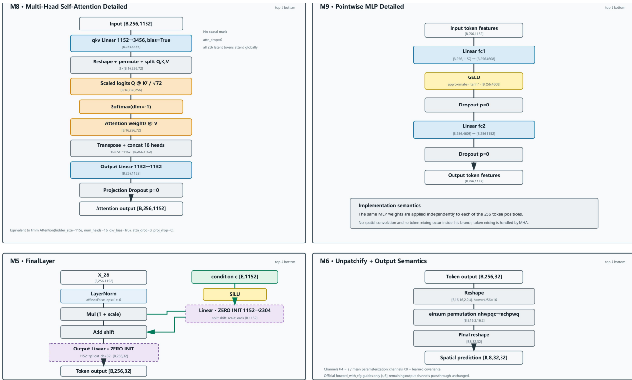
Figure A4 局部放大：最新版 M8 Multi-Head Self-Attention、M9 Pointwise MLP、M5 FinalLayer 与 M6 Unpatchify/输出语义。
