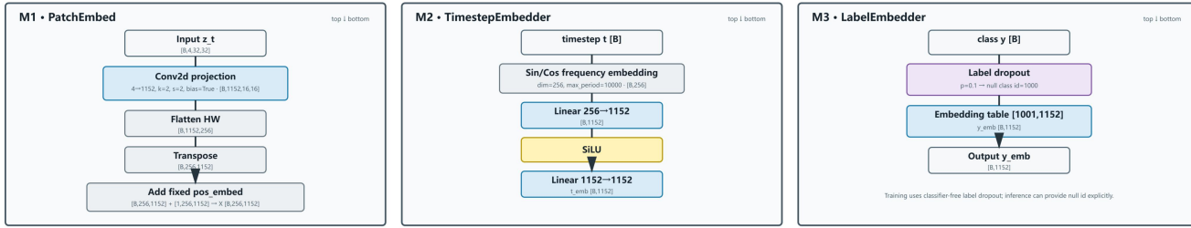
Figure A2 局部放大：最新版 M1 PatchEmbed、M2 TimestepEmbedder 与 M3 LabelEmbedder，包含逐层运算和 tensor shape。
