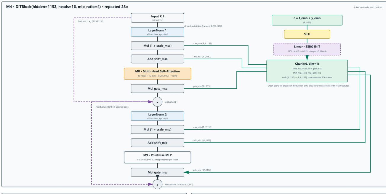
Figure A3 局部放大：最新版 M4 DiTBlock，完整展示 adaLN-Zero 六路 modulation、attention/MLP 主轴、condition broadcast 与两条 residual bypass。
