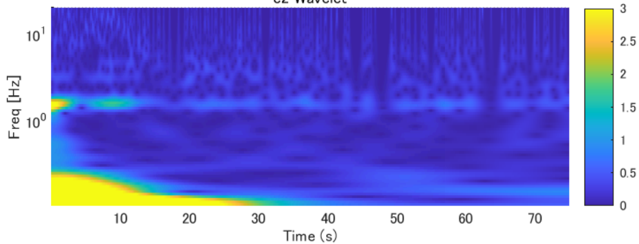
e2 Wavelet
