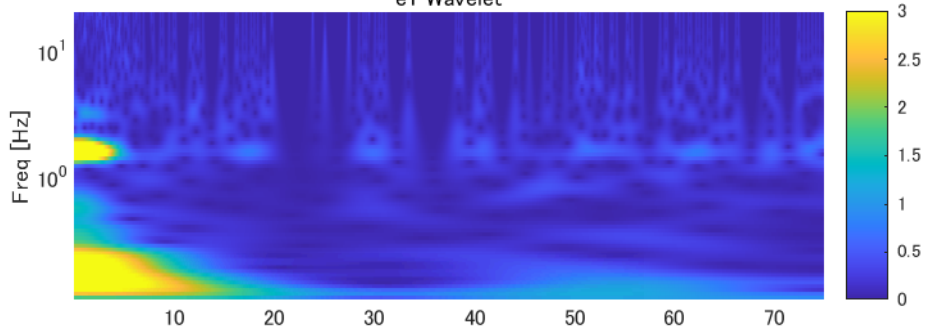
e1 Wavelet
