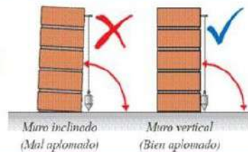
Supervisar con la plomada la verticalidad de los muros
