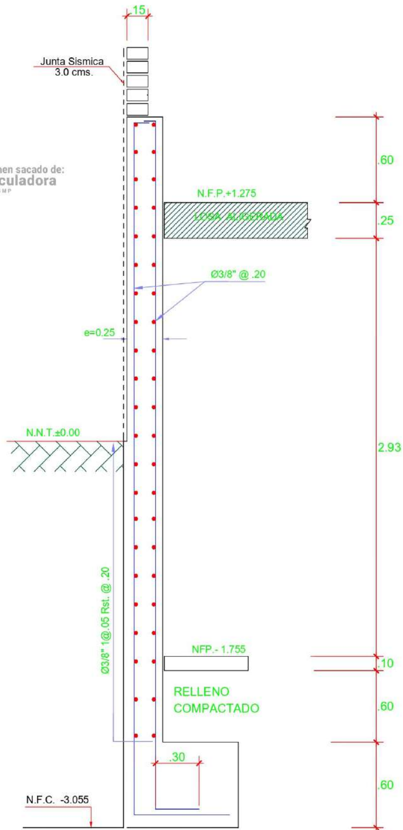
CORTE DE MURO - CORTE 1-1
