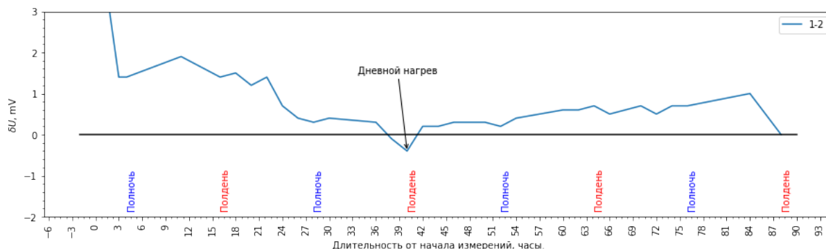
Рис. 13: Разность потенциалов пары собранных медно-сульфатных неполяризуемых электродов с каолином в картонно-тканевых ячейках.
