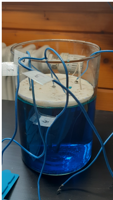
Рис. 8: Медные электроды в насыщенном растворе \text{CuSO}_4
