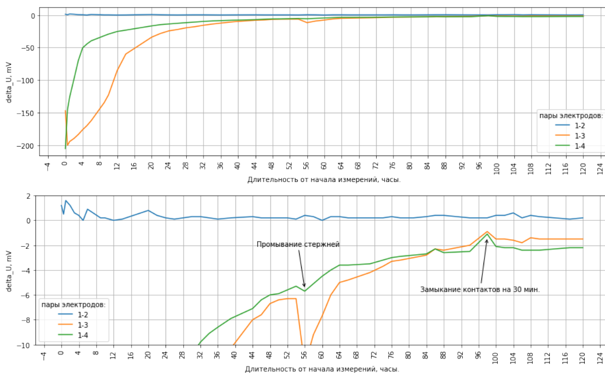
Рис. 16: Изменение разности потенциалов графитовых электродов №1, №2, №3, №4 в растворе сульфата меди. Повторный эксперимент. 1) Полный диапазон измерений (до -200 мВ) 2) В диапазоне от -10 до +2 мВ.
