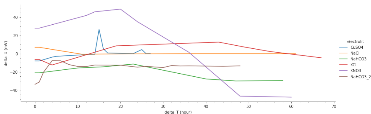
Рис. 15: Изменение разности потенциалов графитовых электродов №1, №2 в растворах разных электролитов. Первый эксперимент.
