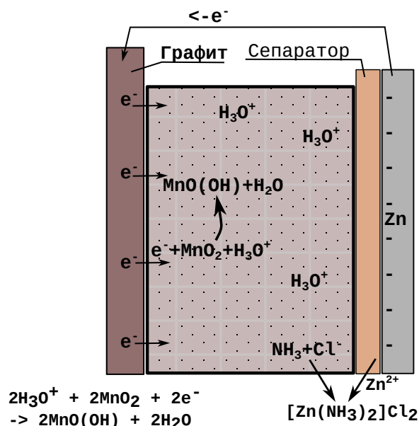
Рис. 7: Процессы в элементе Лекланше при замыкании цепи
