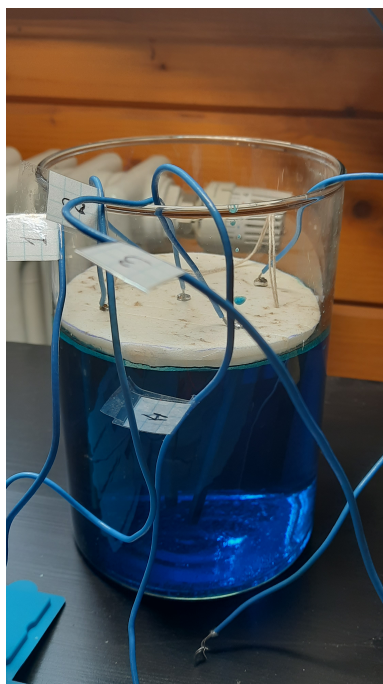
Рис. 8: Медные электроды в насыщенном растворе CuSO_4
