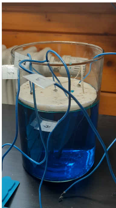
Рис. 8: Медные электроды в насыщенном растворе \text{CuSO}_4
