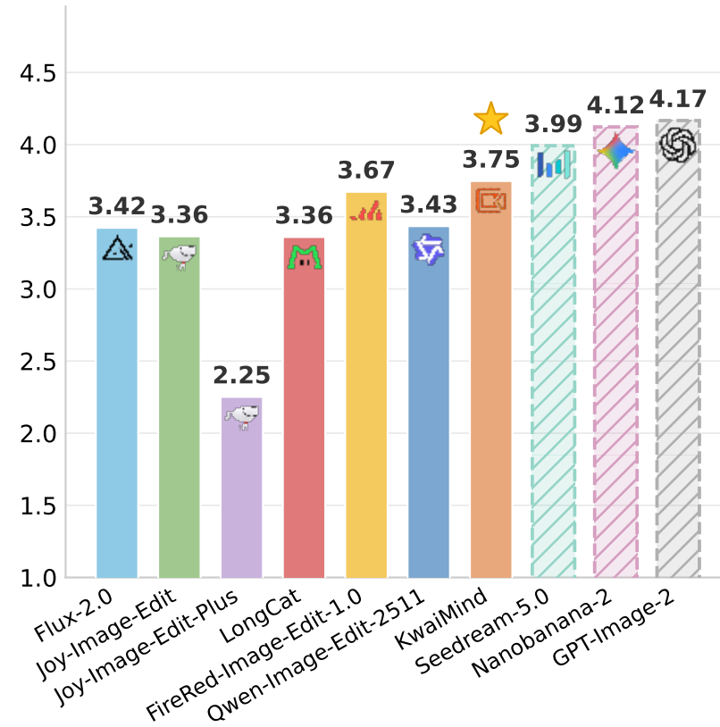
REDEdit (EN)
