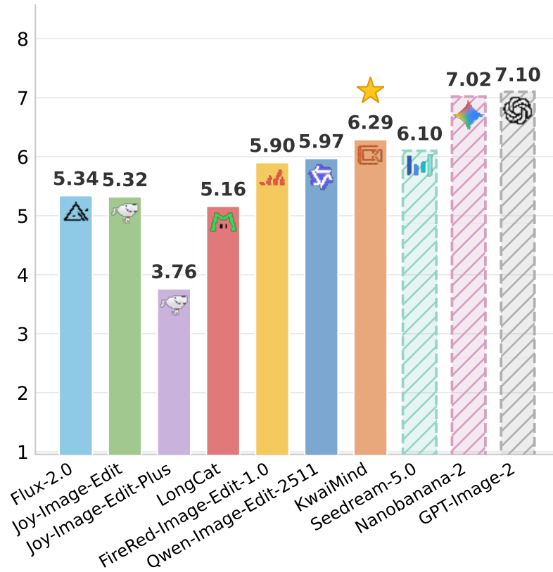
GEEdit (Gemini)
