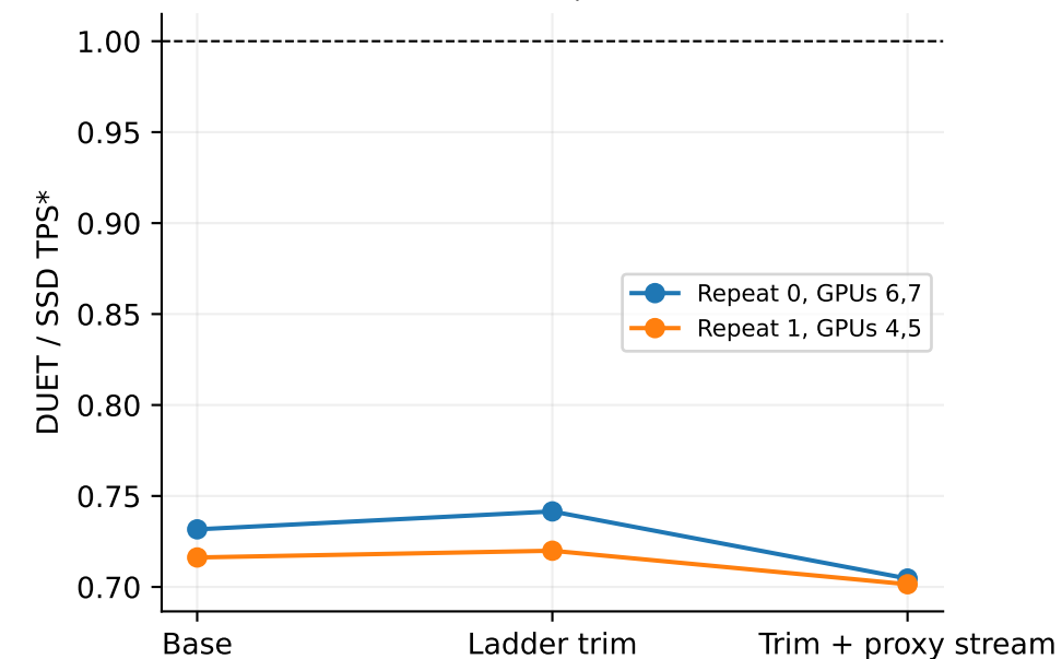
LLAMA3, B=8
