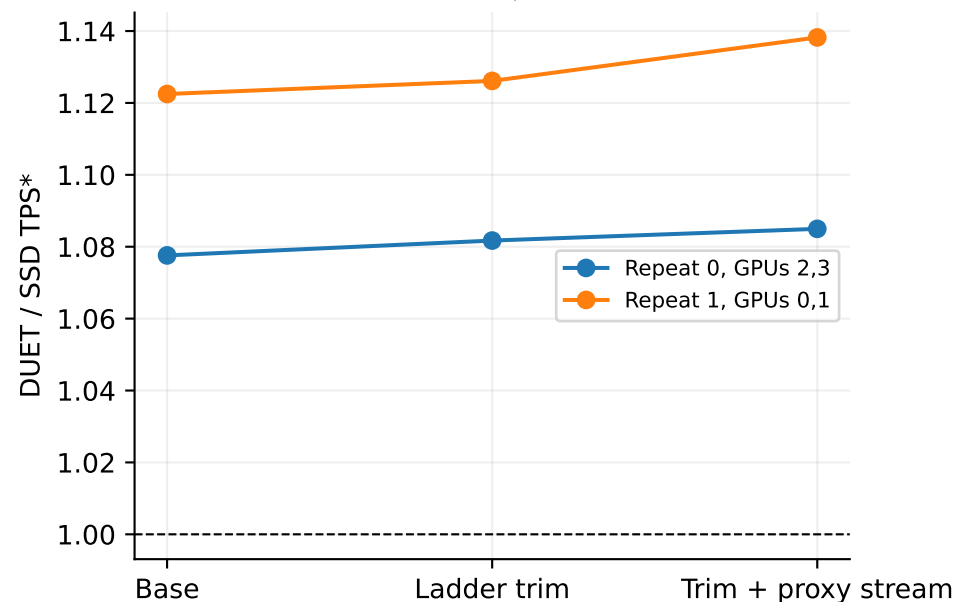
LLAMA3, B=1
