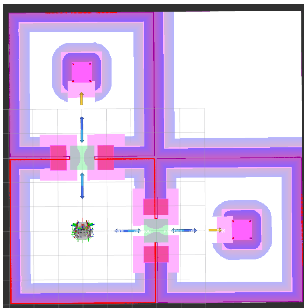
Slika 6.4. Ploha cijene izvedena iz karte: zabranjujuća jezgra oko stolova i zidova, trake nulte cijene kroz prolaze i prilazne poze (plave strelice)
