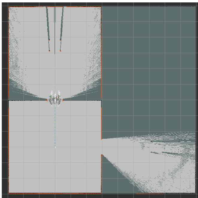
Slika 6.2. Izgradnja karte u tijeku: soba HOME (dolje lijevo) je snimljena, a robot iz prolaza vidi crvenu sobu (gore) i kroz drugi prolaz dio plave (desno); tamno sivo je još neistraženi prostor. Orijentacija je ista kao na slici 6.3
