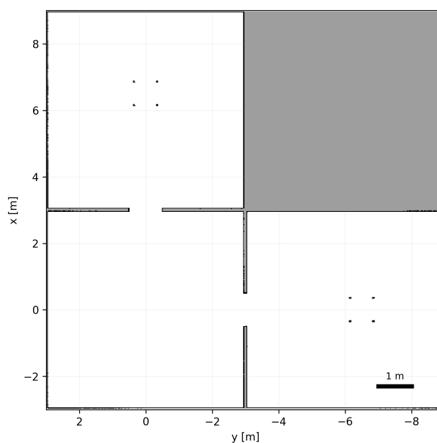
Slika 6.3. Izgrađena karta razlučivosti 0,02 m: 103,9 m 2 slobodne površine na rasponu 11,9 × 11,9 m
