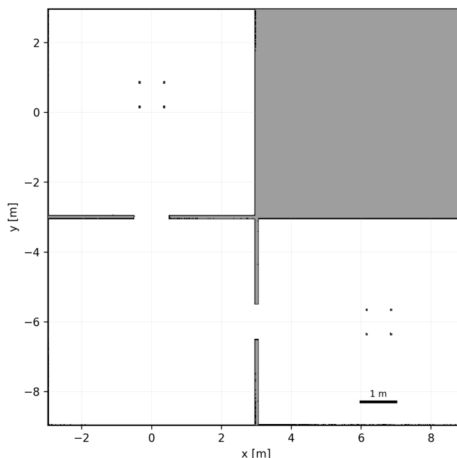
Slika 6.2. Izgrađena karta razlučivosti 0,02 m: 103,9 \text{ m}^2 slobodne površine na rasponu 11,9 \times 11,9 m
