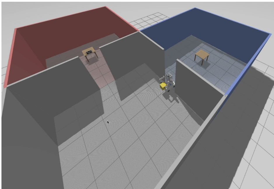
Slika 6.1. Sustav u radu: robot nosi kutiju iz plave sobe kroz prolaz prema crvenoj, u kojoj je na stolu odredišni marker. Vožnja se izvodi na unaprijed izgrađenoj karti, uz lokalizaciju umjesto SLAM-a
