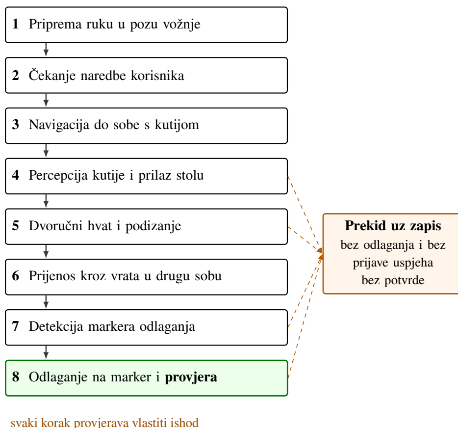
Slika 8.1. Koraci misije; svaki korak provjerava vlastiti ishod, a neuspjeh vodi u prekid uz zapis razloga umjesto u nastavak
