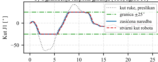
b) Ograničenje raspona gibanja (T3b, zglob J1)
