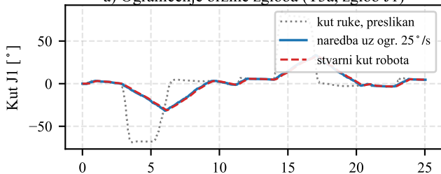
a) Ograničenje brzine zgloba (T3a, zglob J1)
