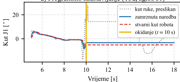
d) Programsko zaustavljanje (T3d, zglob J1)
