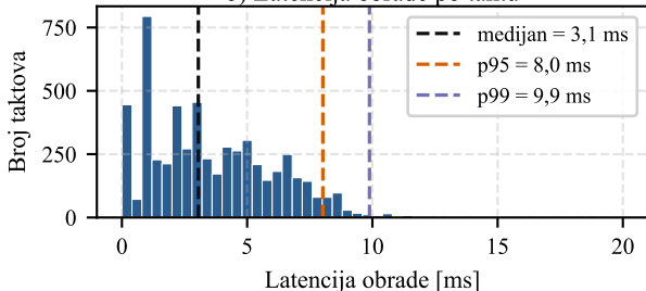
b) Latencija obrade po taktu
