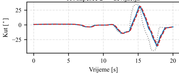
J5: zapešće 2 — devijacija
