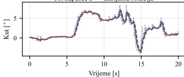
J6: zapešće 3 — aksijalna rotacija
