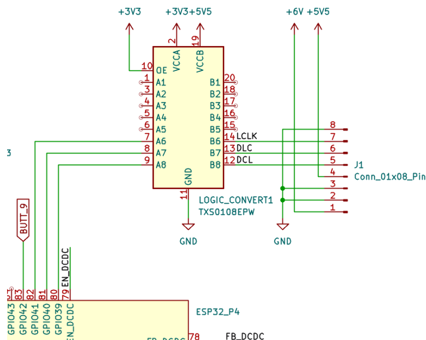
Obrázek 4.13: Zapojení převodníku logických úrovní pro komunikaci s objektivem v eschématu. [Zdroj: Vlastní]
