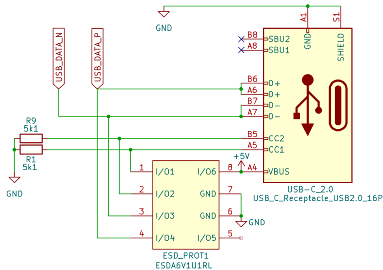
Obrázek 4.14: Zapojení USB-C konektoru v eschématu. [Zdroj: Vlastní]
