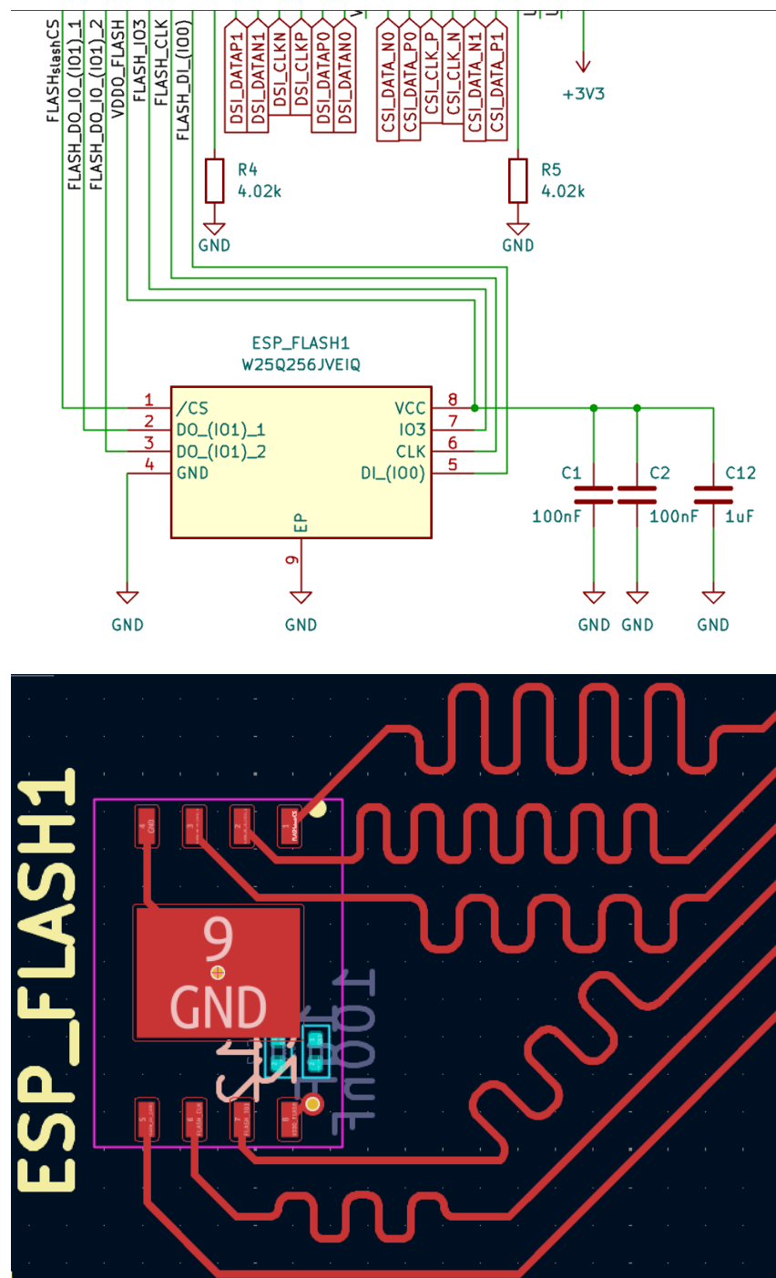
Obrázek 4.7: Zapojení externí flash paměti v eschématu a v PCB editoru. [Zdroj: Vlastní]
