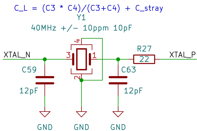
Obrázek 4.12: Zapojení externího krystalu v eschématu. [Zdroj: Vlastní]
