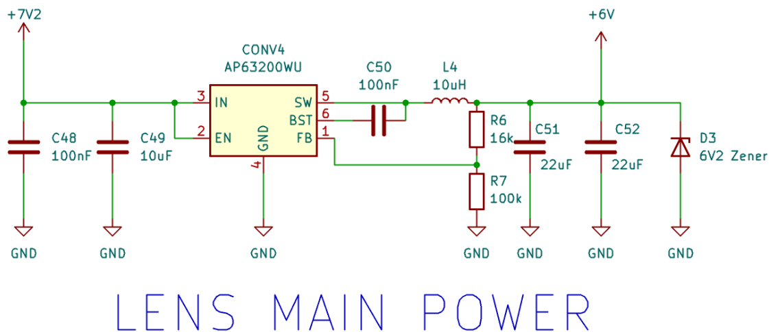
Obrázek 4.6: Zapojení měniče napětí pro obsluhu servo motorů v objektivu [Zdroj: Vlastní]
