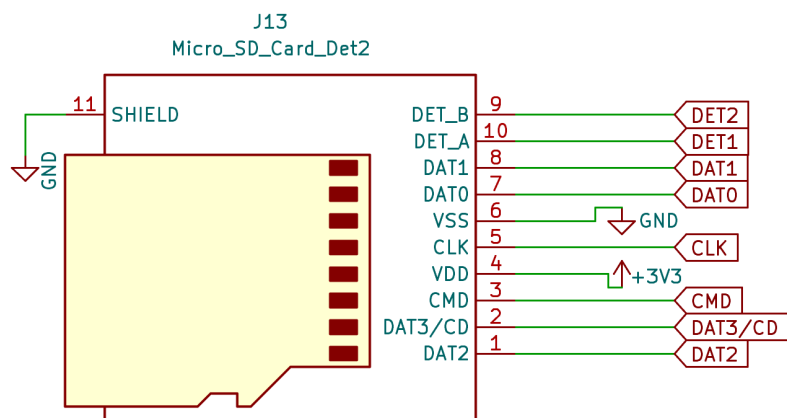
Obrázek 4.11: Zapojení slotu pro SD kartu v eschématu. [Zdroj: Vlastní]
