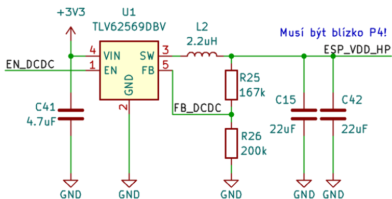
Obrázek 4.2: Schémata zapojení měniče pro napájení HP pinů [Zdroj: Vlastní]
