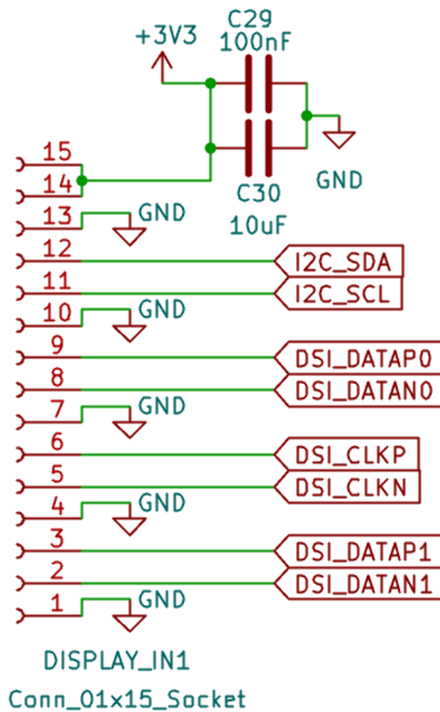
Obrázek 4.10: Zapojení konektoru pro připojení displeje v eschématu. [Zdroj: Vlastní]
