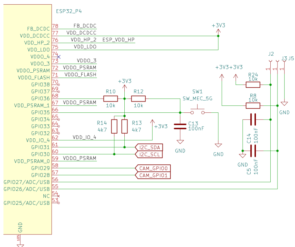
Obrázek 4.3: Zapojení kolem ESP32-P4 popsané v této sekci: I2C pull-upy, reset a startovací vazby. [Zdroj: Vlastní]
