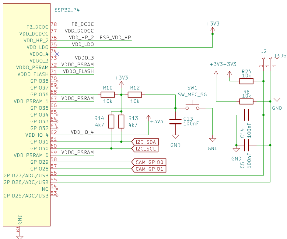
Obrázek 4.3: Kritické pomocné zapojení kolem ESP32-P4: I2C pull-upy, reset a startovací vazby. [Zdroj: Vlastní]
