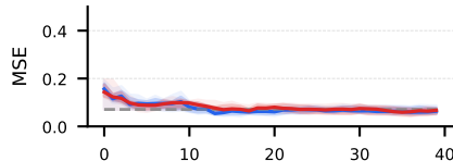
MSE
