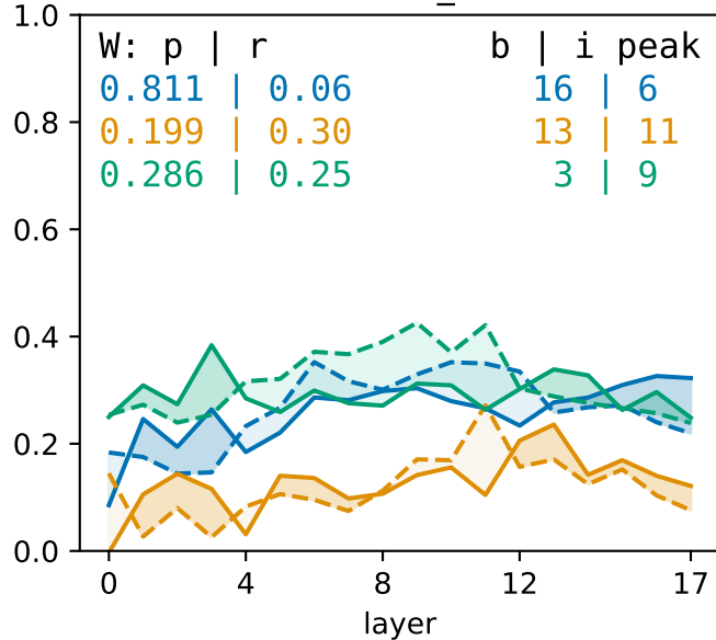
Gemma_2B
