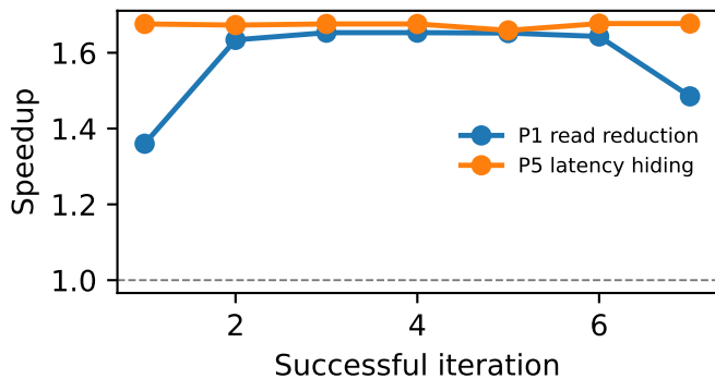
Softmax A
