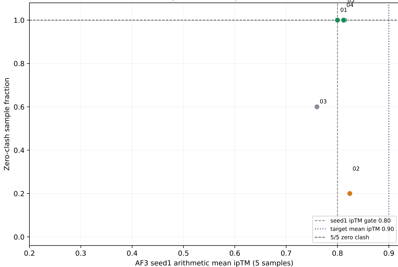
E299 E292-parent clash repairs: AF3 seed1
