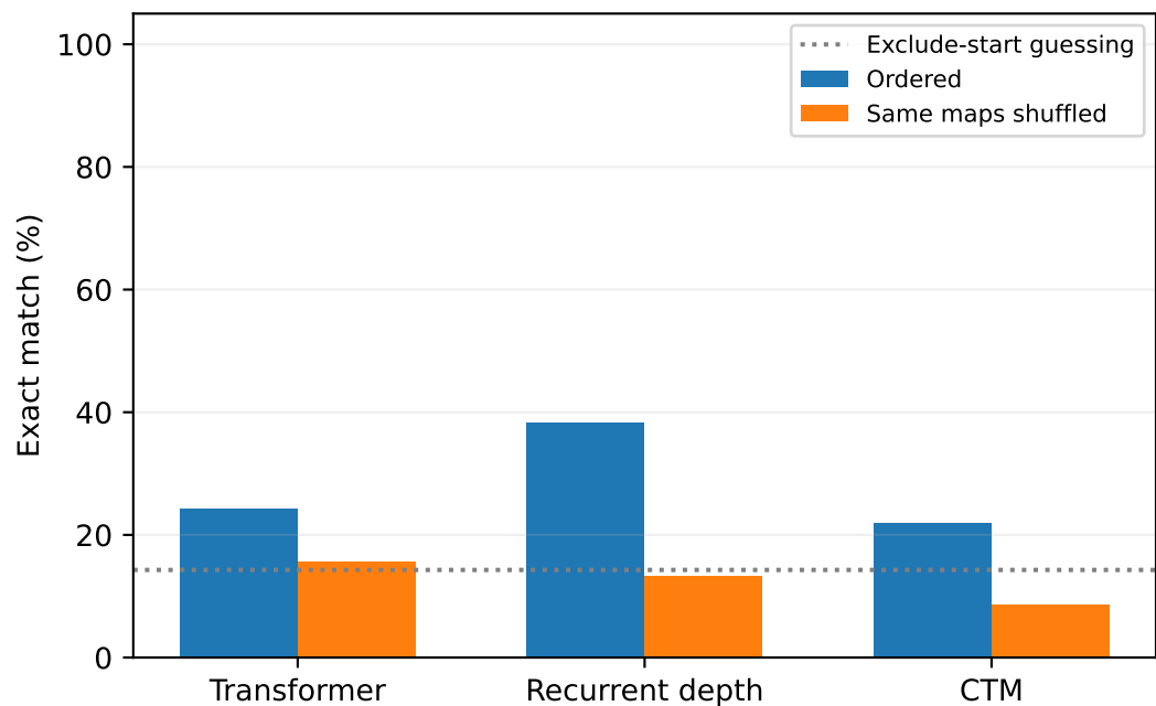
Paired held-out evaluation
