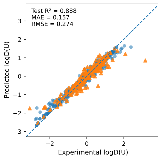
AdaBoost
