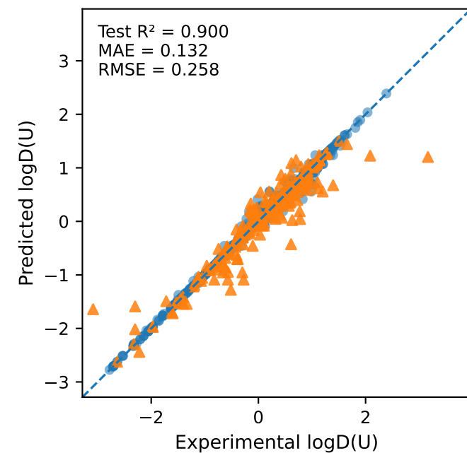
MLP
