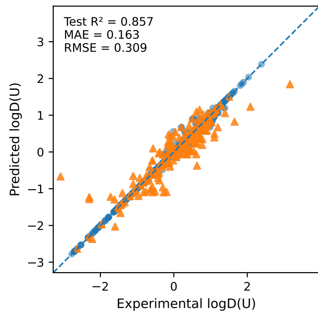
GradientBoosting
