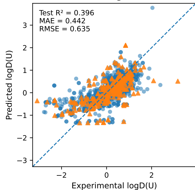
KNN
