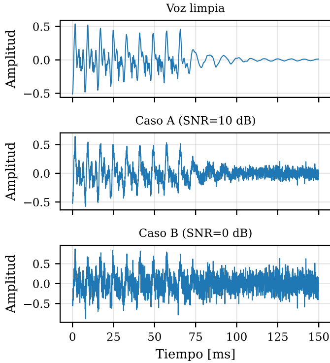
Figura 2: Comparación temporal de la voz limpia, Caso A (SNR = 10 dB) y Caso B (SNR = 0 dB) durante 150 ms de habla activa.
