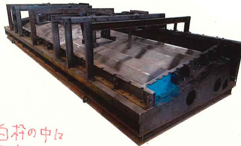
◆ 幕墙板模具构件
