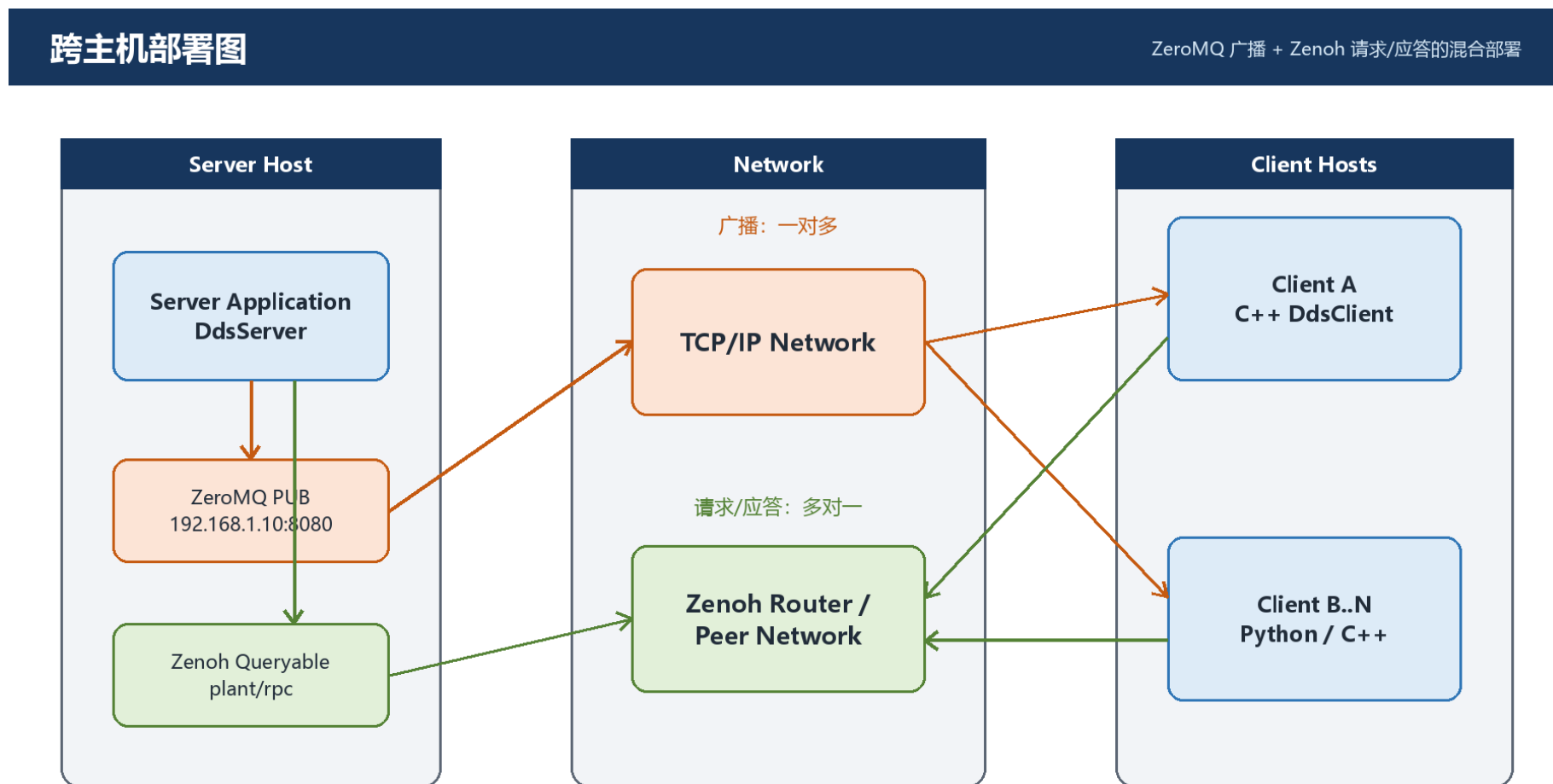
图 7 跨主机部署图
