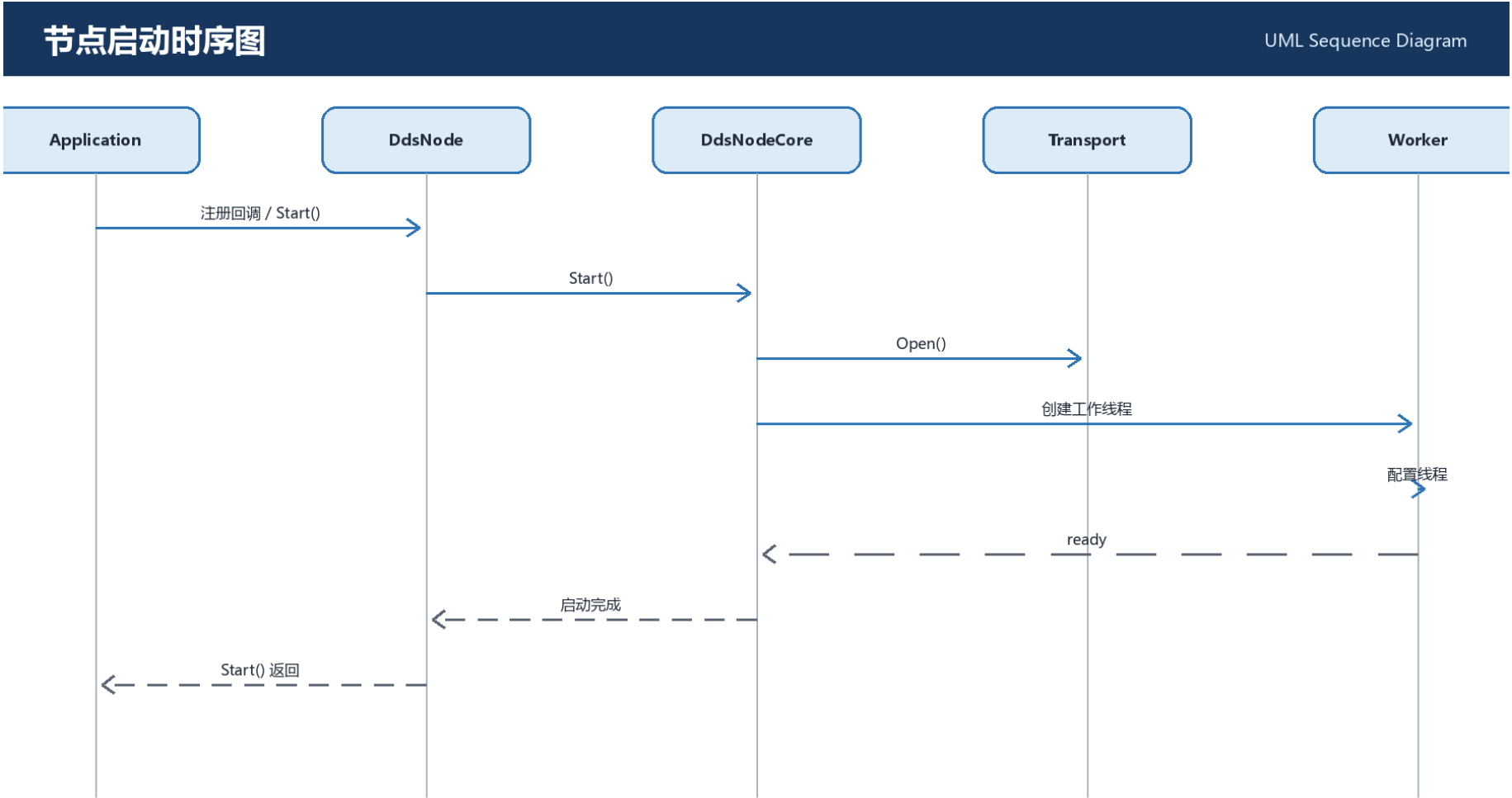
图 4 节点启动时序图
