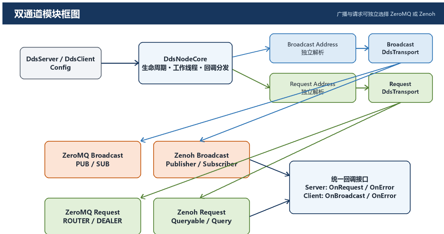
图 2 双通道模块框图
