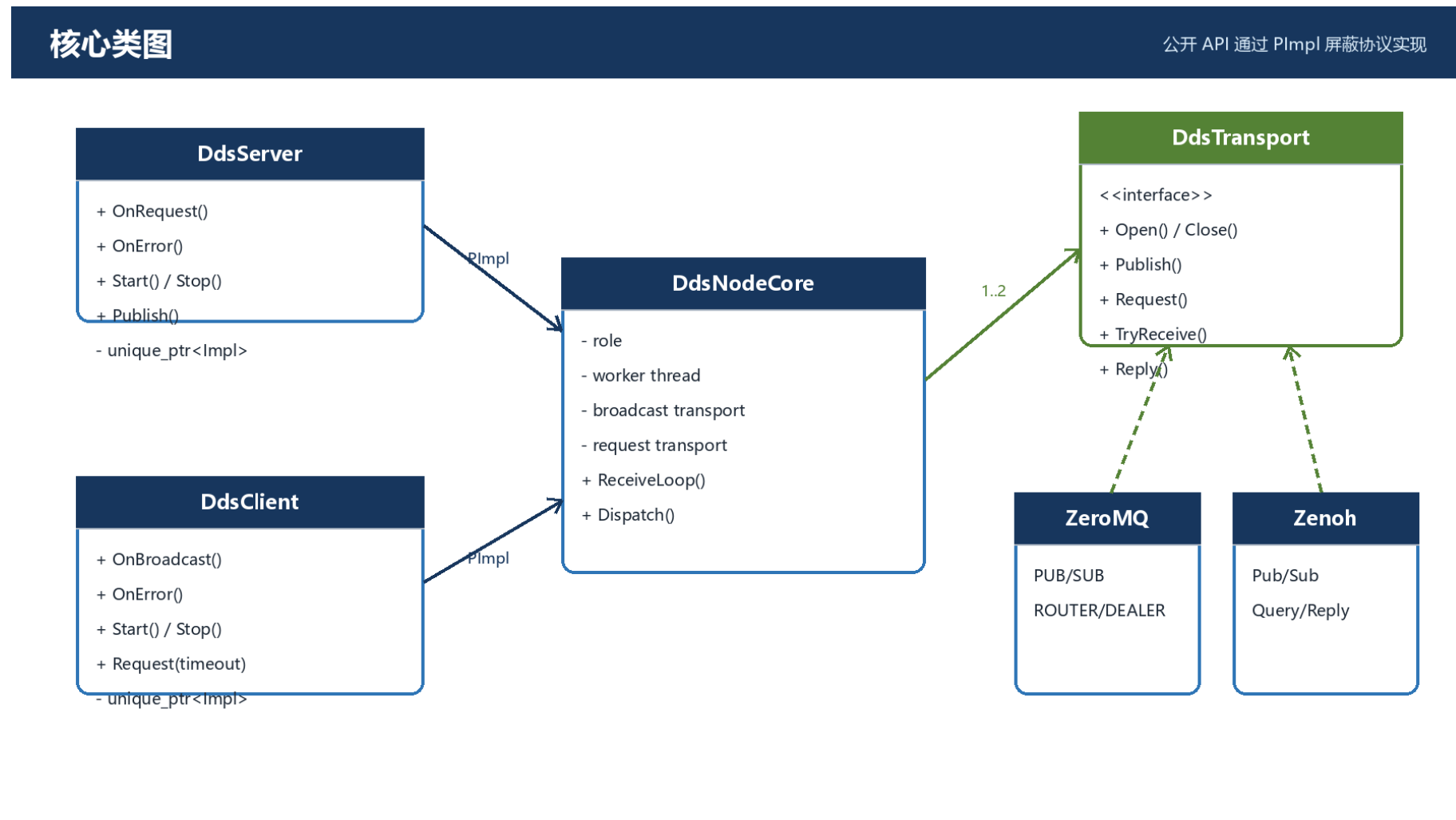
图 3 核心类图
