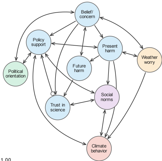
B Example FCI PAG
