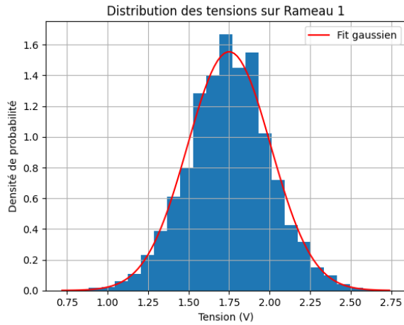
(a) Fit gaussien des mesures de Rameau 1 (densité de probabilité)
