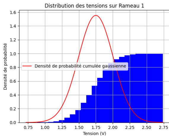
(a) Densités de probabilités cumulatives des mesures de Rameau 1
