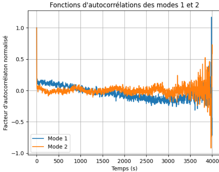
FIGURE 12 – Facteur d'autocorrélation des modes 1 et 2 en fonction du temps.
