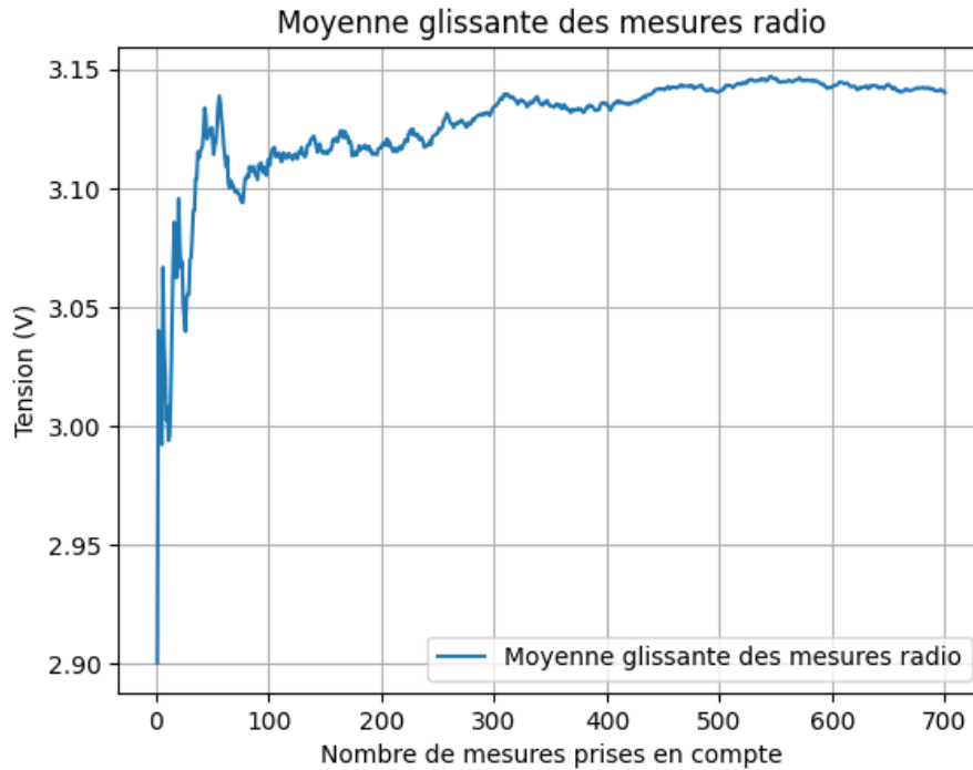
FIGURE 16 – Evolution de la moyenne expérimentale en fonction du nombre de mesures
