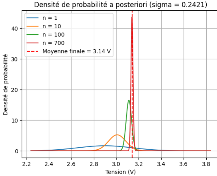
FIGURE 18 – Densité de probabilité à posteriori de la tension v pour n mesures
