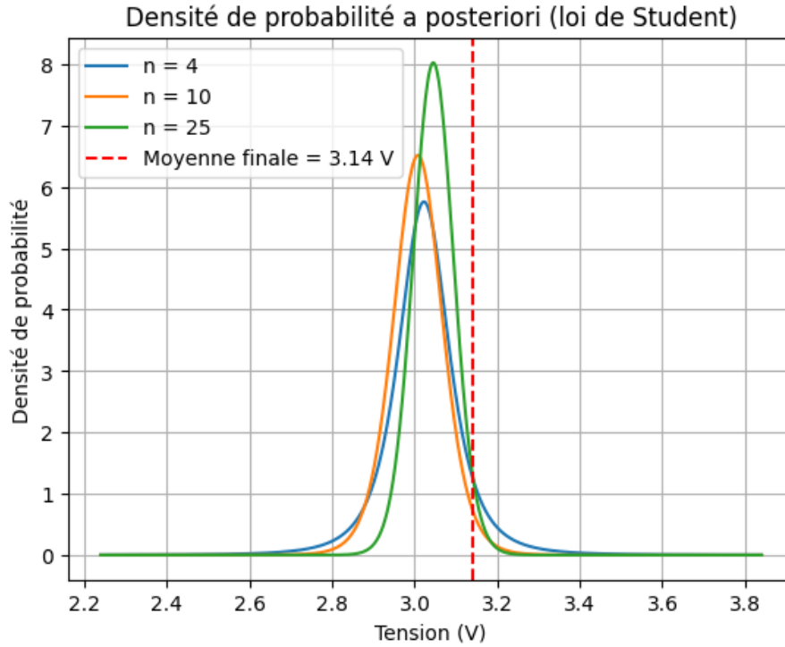
FIGURE 19 – Densité de probabilité à posteriori de la tension v pour n mesures ne connaissant pas la précision expérimentale
