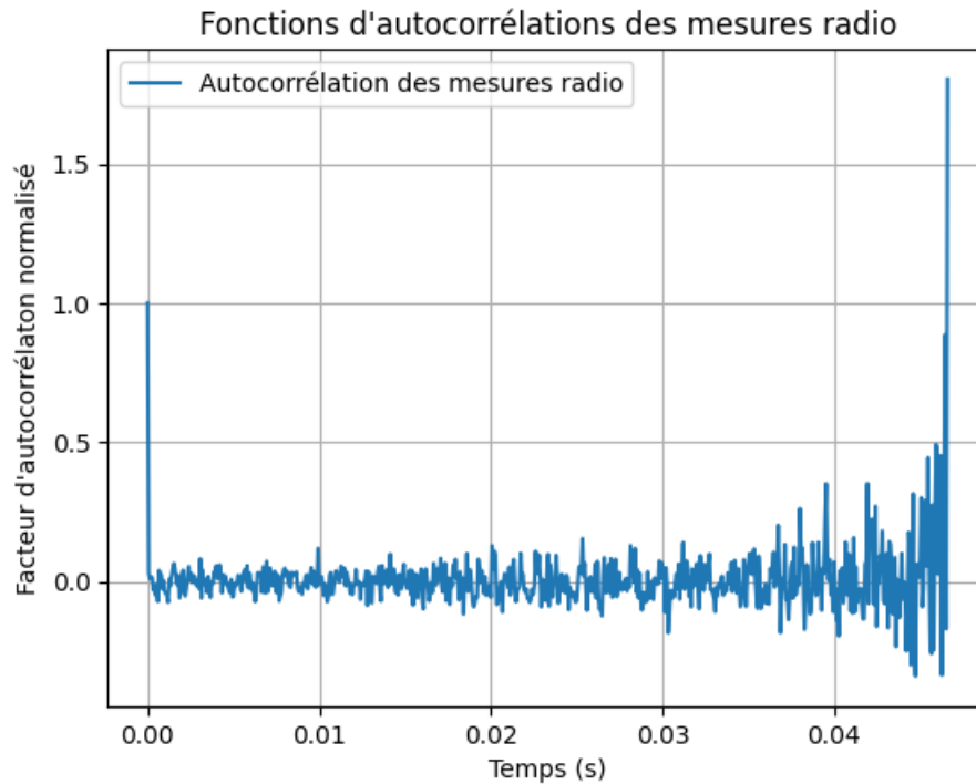
FIGURE 15 – Fonction d'auto-corrélation des mesures radios par Rameau
