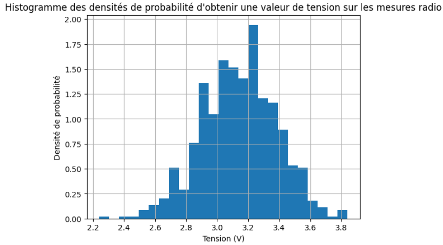
FIGURE 14 – Histogramme des densités de probabilité d'obtenir une valeur de tension sur les mesures radio
