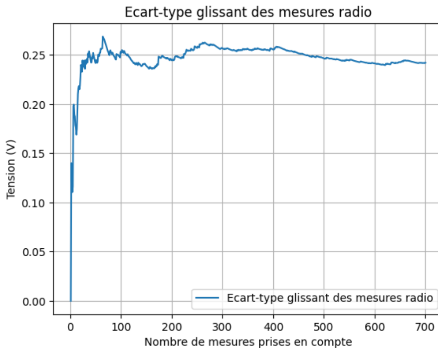
FIGURE 17 – Evolution de l'écart-type expérimental en fonction du nombre de mesures
