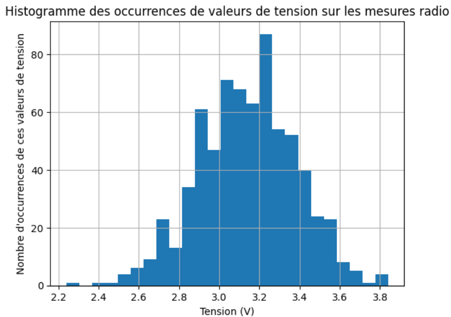
FIGURE 13 – Histogramme des occurrences de valeurs de tension sur les mesures radio
