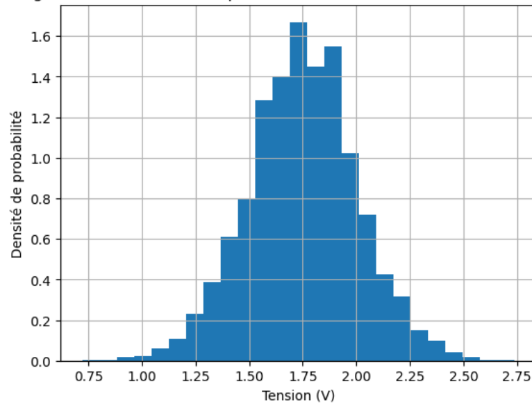
FIGURE 5 – Densité de probabilité d'obtenir une valeur de tension pour Rameau 1
