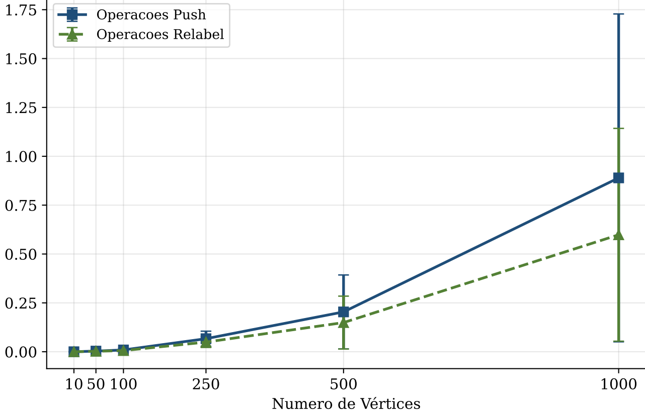
Operações Push e Relabel vs Tamanho da Rede
