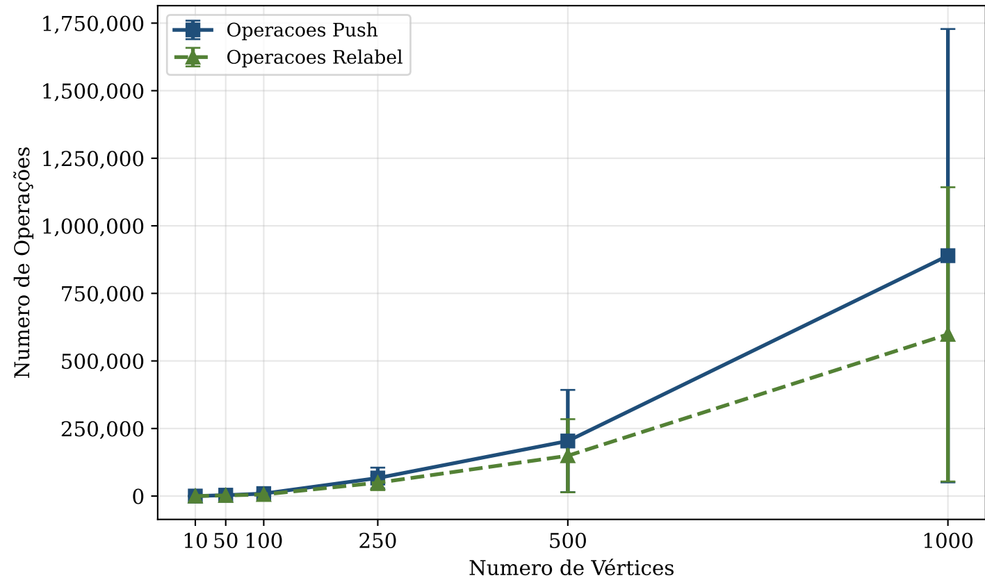
Operações Push e Relabel vs Tamanho da Rede
