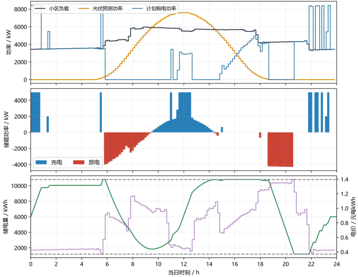
图 5-1 问题 1 购电与储能调度结果
