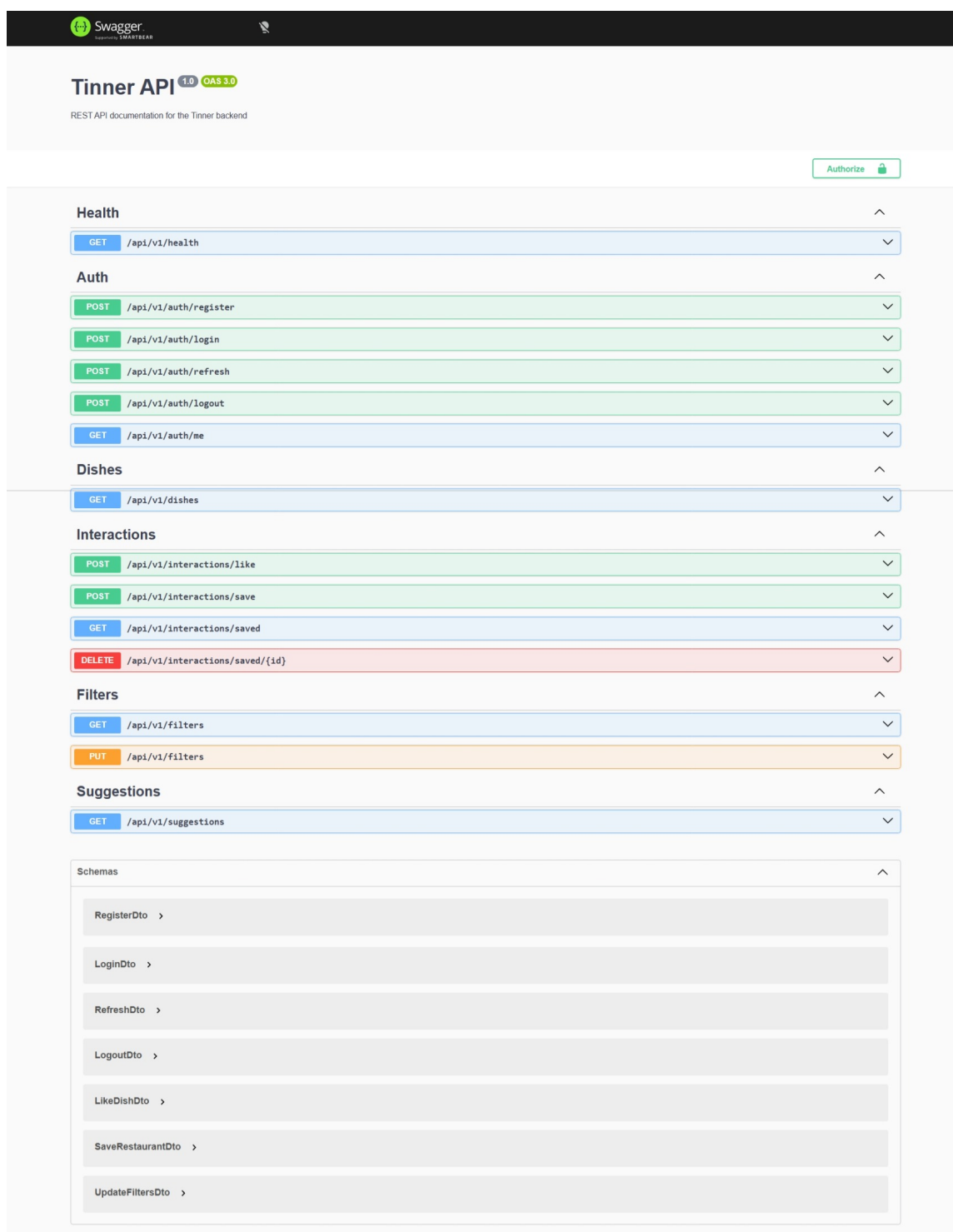
Hình 8: Giao diện tài liệu hóa API tự động qua NestJS Swagger UI phục vụ tích hợp
