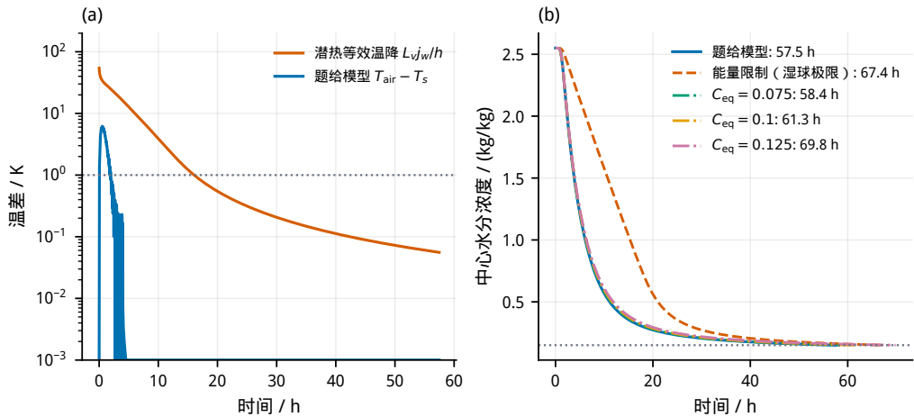
图 14 模型评价扩展: (a) 题给模型蒸发率所对应的潜热等效温降 L_v j_w / h 与模型实际的表面温差 T_{\text{air}} - T_s (纵轴对数坐标, 点线为 1 K) ——前十余小时前者远大于后者, 说明题给能量方程未支付蒸发潜热; (b) 题给模型、能量限制情形与三档平衡含水率驱动力下的中心水分浓度时程, 点线为判据 0.15 \text{ kg}/\text{kg} 。图 (a) 中模型温差在 2–4 h 间因烘房温度样本的 \pm 0.3^\circ\text{C} 噪声而在零附近改变符号, 负值在对数坐标下被截断, 故呈现振荡带。
