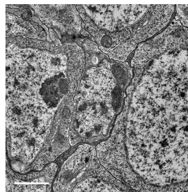
C BA1c SU Neuron
